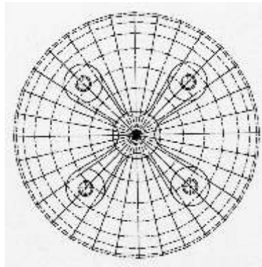
Punktgehaltene Kunststoffverglasung B1 Punkthalter aus Aluminiumguss in Eigenentwicklung
